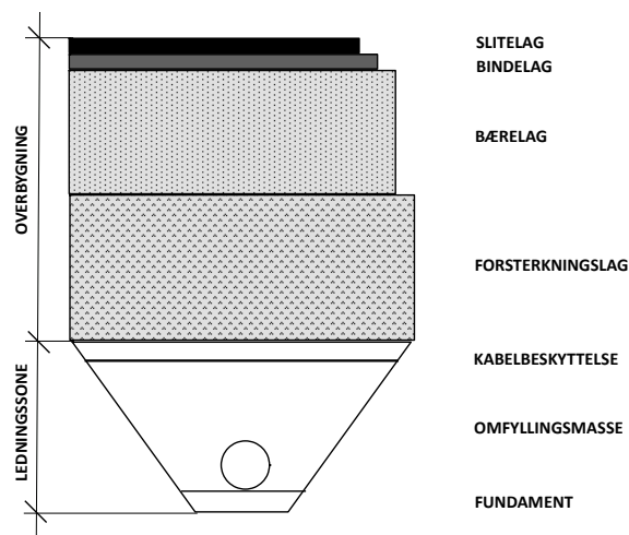
Figur 3: Ledningssonen plasseres under vegoverbygningen
