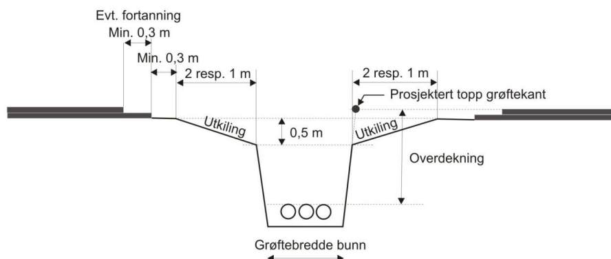
Figur 5: Utkiling for å hindre setninger ved dype kryssende grøfter.
